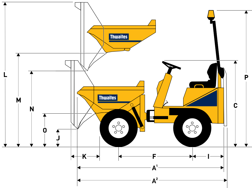
Dimensiones (mm)
